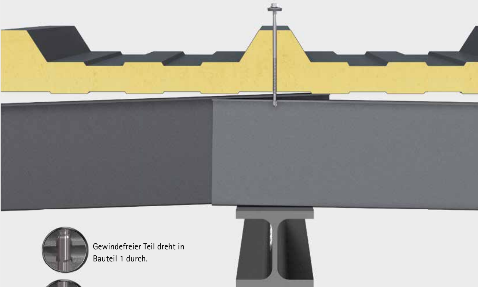
Bohrspitze bohrt sich währenddessen durch Bauteil 2.
